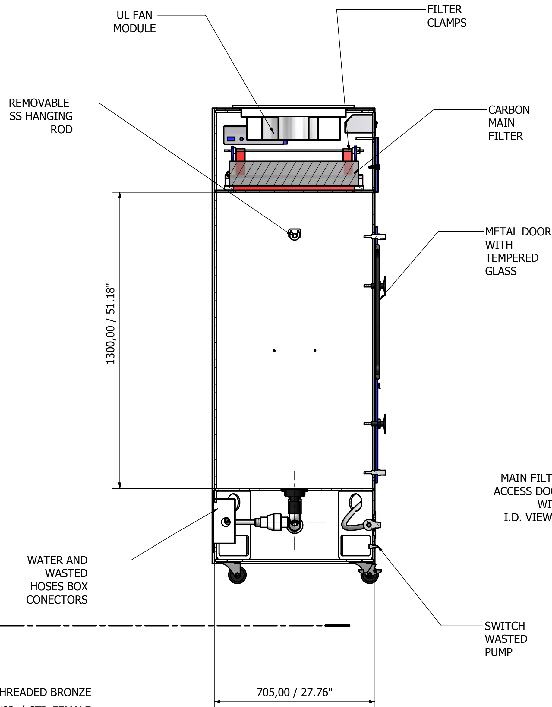
A-A ( 1 : 10 )
